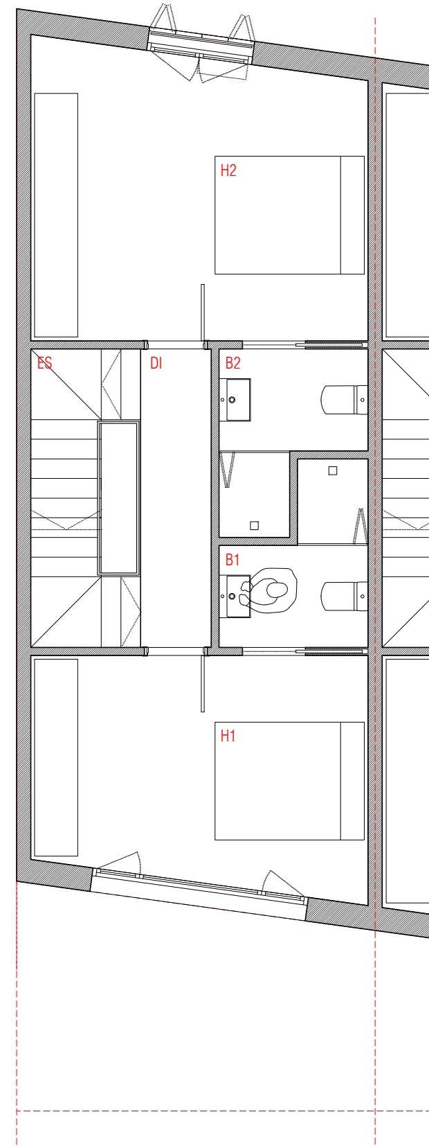
PLANTA 1ª_1/75
