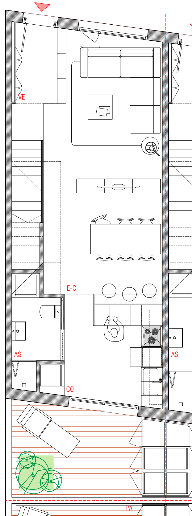
PLANTA BAJA_1/75
