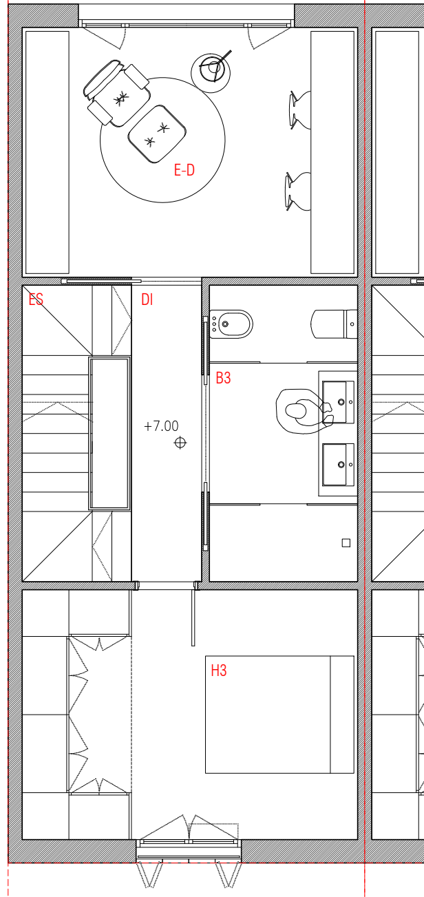
PLANTA 2ª_1/75
