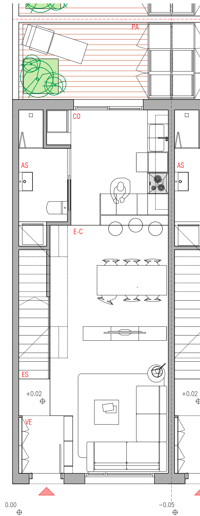
PLANTA BAJA_1/75
