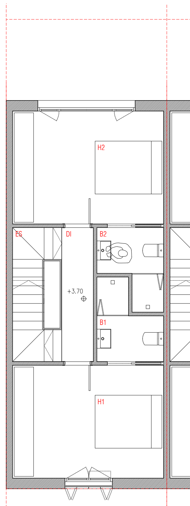
PLANTA 1ª_1/75
