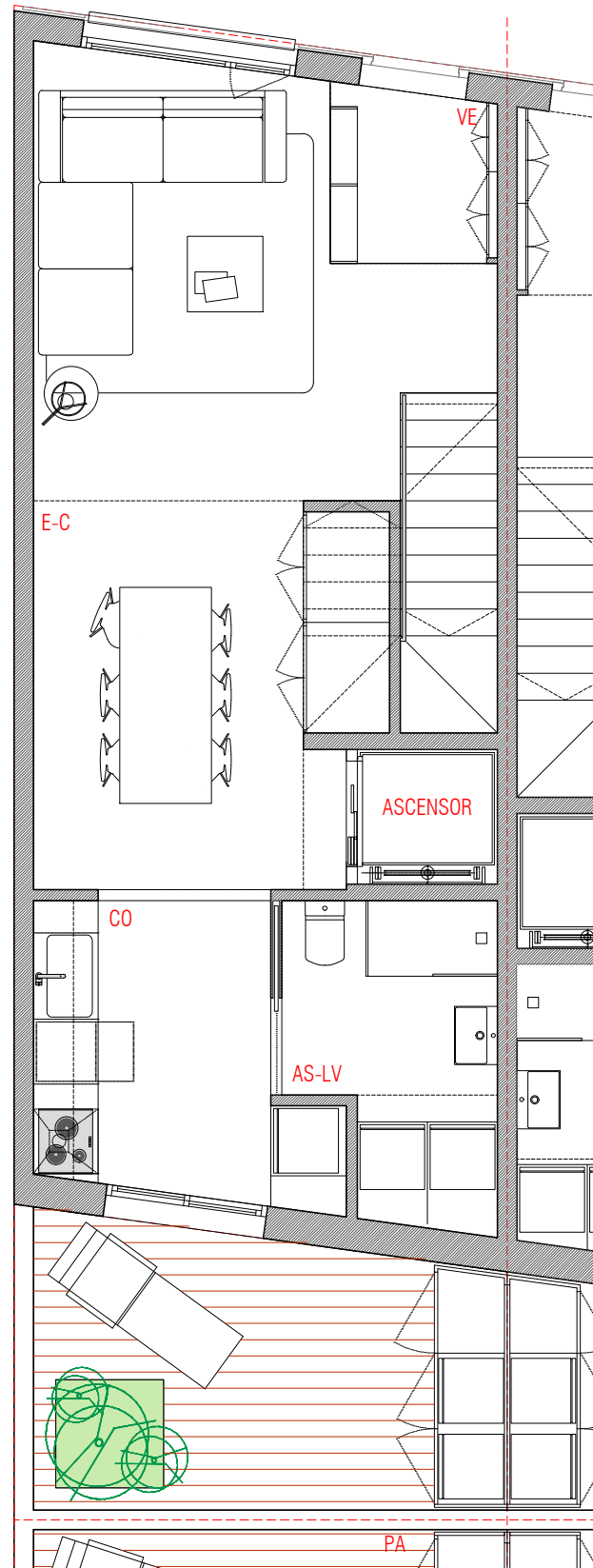
PLANTA BAJA_1/75
